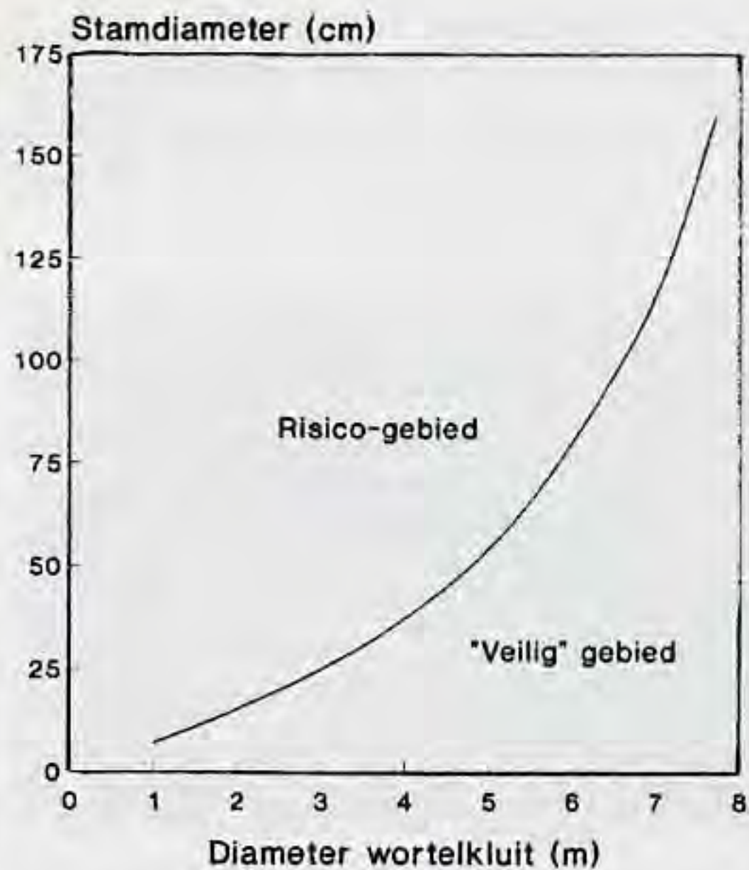
Figuur 1: Een zgn. windworpdiaagram waarin de minimale verhouding tussen de noodzakelijke diameter van de wortelkluit in relatie tot de boomgrootte (uitgedrukt in stamdiameter) is aangegeven (naar: Mattheck & Breloer, 1995).
